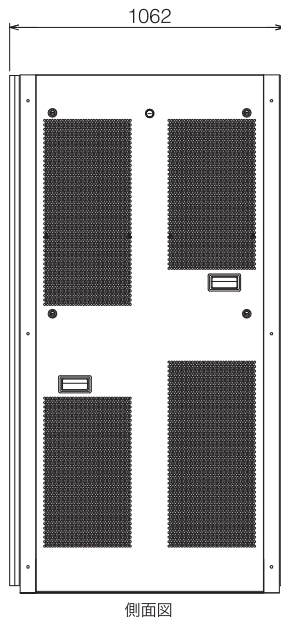
側面図
